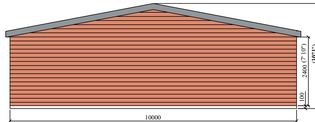
END ELEVATION
